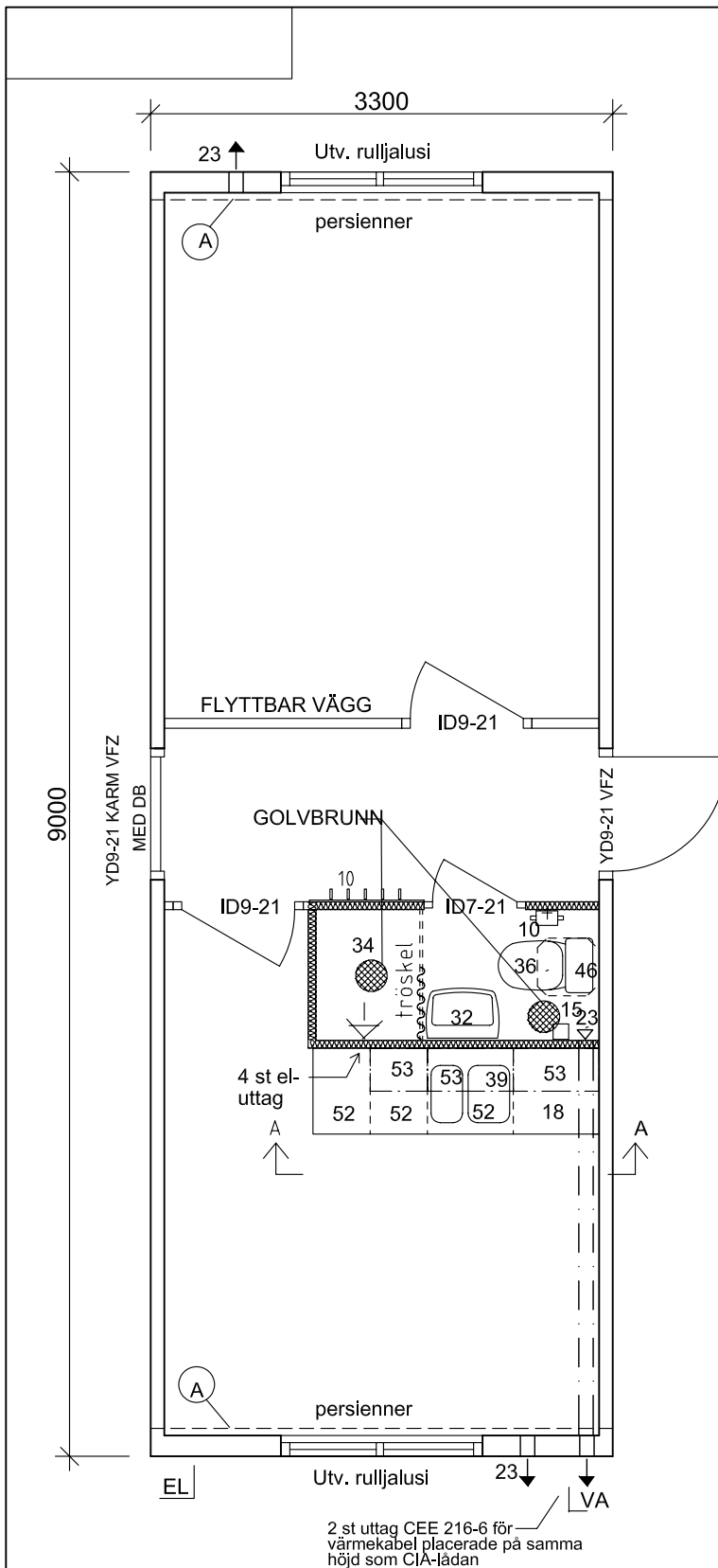
Inrede A-A
